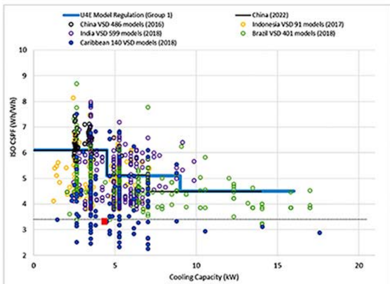
Figure 12: Efficacité en ISO CSPF estimée pour les CA à vitesse variable disponibles dans certaines économies. Source : PNUE, 2019b. 13 , marque rouge ajoutée par l'auteur pour indiquer la moyenne du Mali pour les CA unitaires à vitesse variable.
