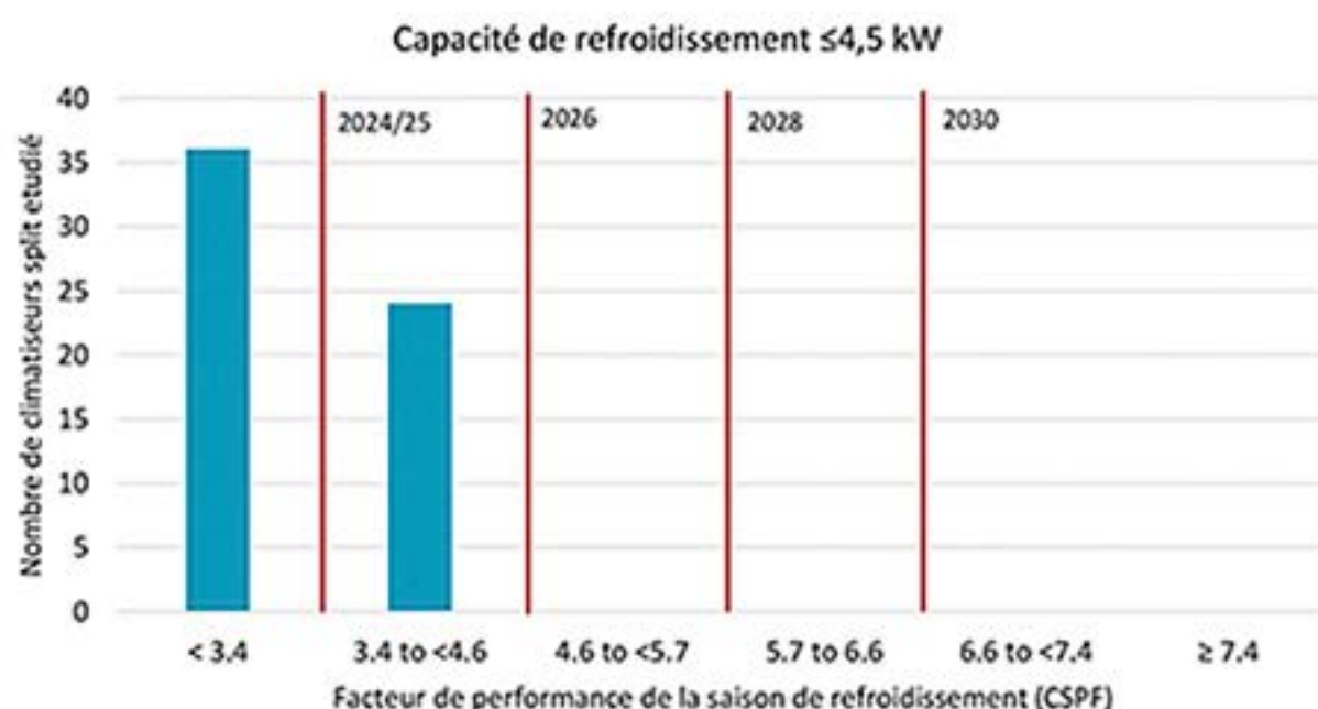
Figure 17: Distribution de fréquence de l'efficacité énergétique des CA étudiés avec une capacité de refroidissement \leq 4,5 kW (sur la base du CSPF estimé pour le groupe climatique 0A), les lignes rouges et les années indiquent les SMPE proposées.
